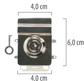
280775.. | Steckschloss 4435
