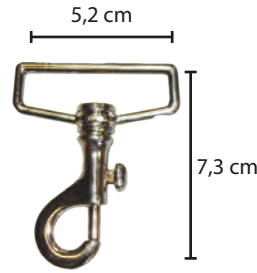
280759.. | Karabinerhaken
