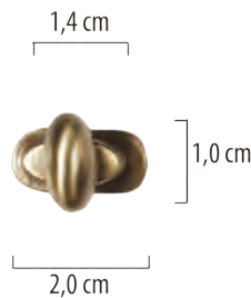
280142.. | Drehverschluss 4722
