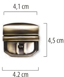
280145.. | Steckschloss 5235
