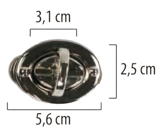
280114.. | Drehverschluss 447K
